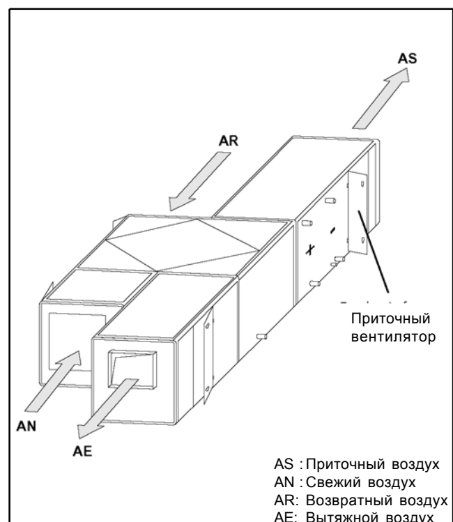
Рис. 3Д - Сторона обслуживания - правая (по отношению к направлению забора свежего воздуха приточным вентилятором)
